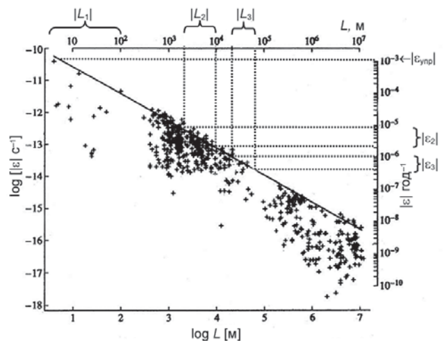
Рис. 1. Распределение модулей скоростей горизонтальных деформаций в зависимости от длины профиля наблюдений с учетом [3]
