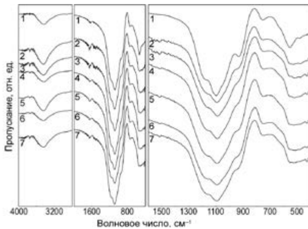
Рис.2. ИК-спектры алюмофосфатных стекол с РЗЭ (1-7 – см. текст)
