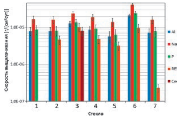
Рис. 3. Скорости выщелачивания элементов из НАФ стекол с добавками оксидов РЗЭ, полученных закалкой расплавов
