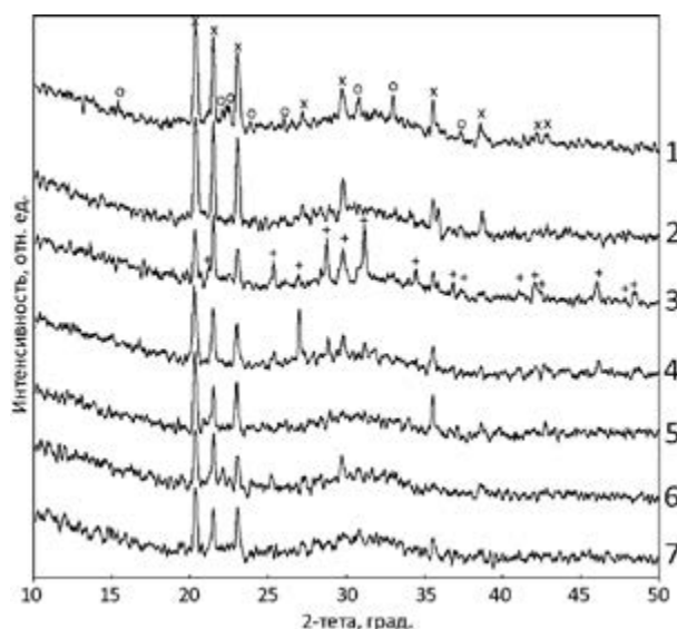
Рис. 1. Рентген-дифрактограммы продуктов, полученных при медленном охлаждении (отжиге) расплавов: × – фосфотридимит, о – β-Na 6 Al 3 (P 2 O 7 ) 3 , + – монацит
