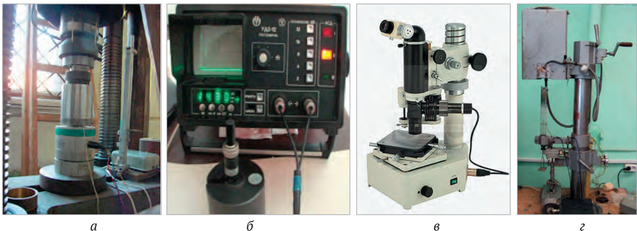
Рис. 2. Фотографии оборудования, на которых проводилось определение основных показателей качества боросиликатных стекол: а — пресс ГМС-50, б — дефектоскоп УД2-12, в — микротвердомер ПМТ-3, г — кварцевый дилатометр-вискозиметр системы Клюева — Черноусова
