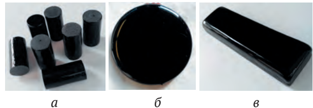
Рис. 1. Фотографии образцов стекол для различных методов испытаний: а — прочность на сжатие и модуль Юнга; б — прочность на изгиб и термостойкость; в — коэффициент линейного термического расширения
