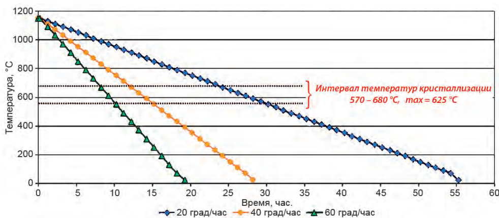
Рис. 5. Температурно-временные режимы проведения опытов по охлаждению расплава БСС-20
