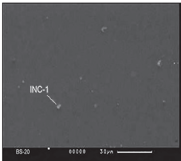
Рис. 6. SEM-микрофотография образца БСС-20, скорость охлаждения 20 °С/ч
