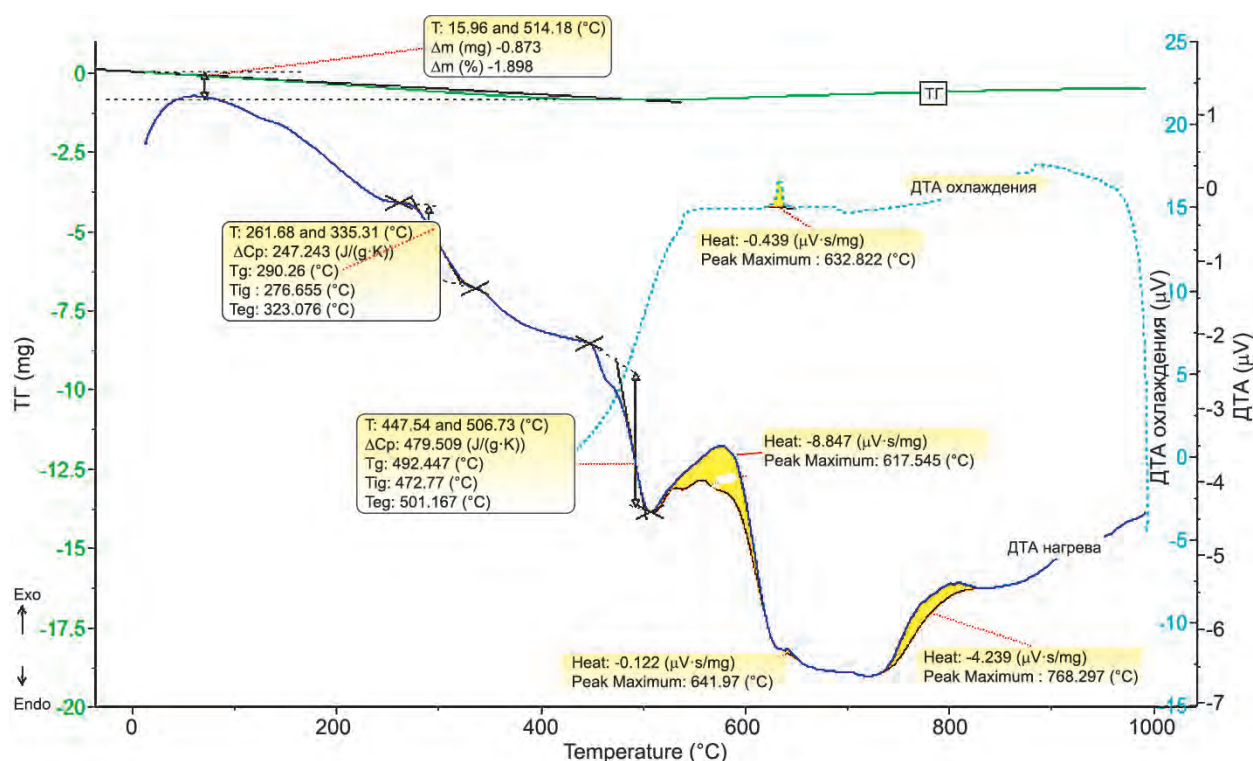
Рис. 3. Дериватограмма образца боросиликатного стекла БСС-20
