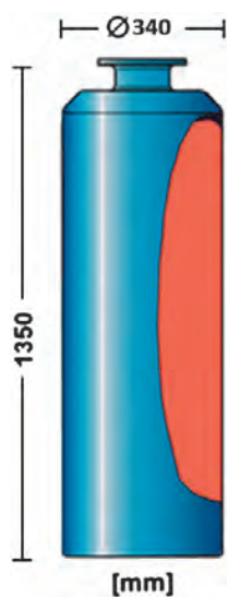
Рис. 4. Общий вид бидона для остеклованных ВАО ОДЦ ГХК ( V \sim 100 \text{ дм}^3 )
